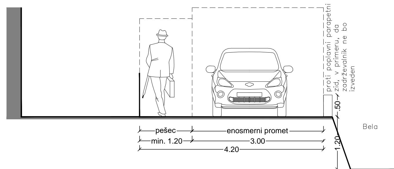
CESTNI PROFIL D-D VAS OD HIŠNE ŠT. 2 DO 4
