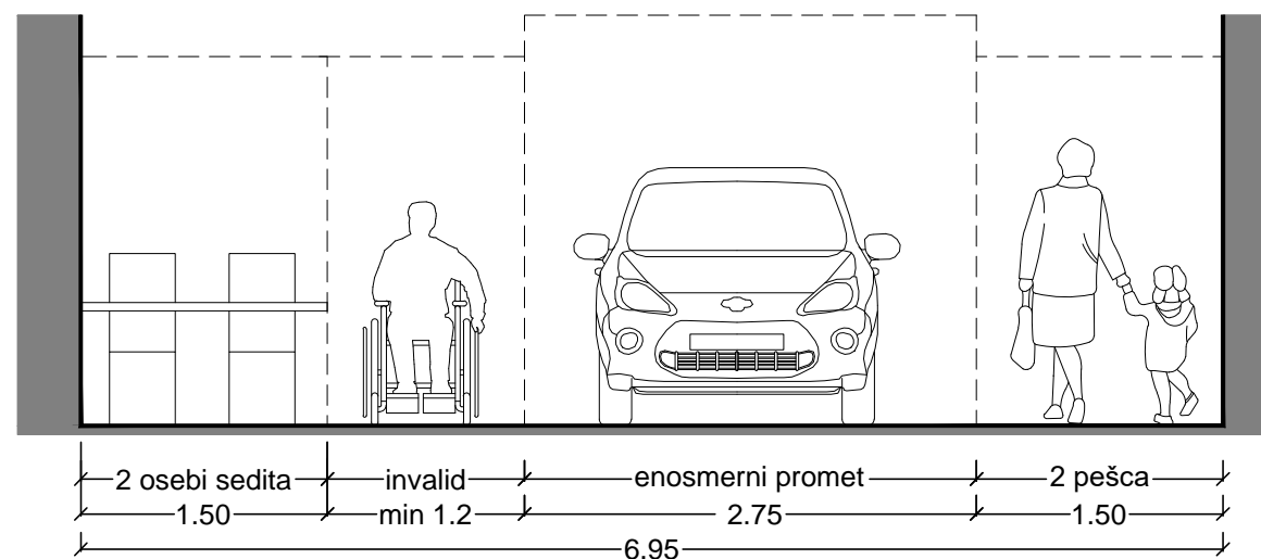
CESTNI PROFIL B-B STARA CESTA OD HIŠNE ŠT. 4 DO 28 IN OD 47 DO 52
