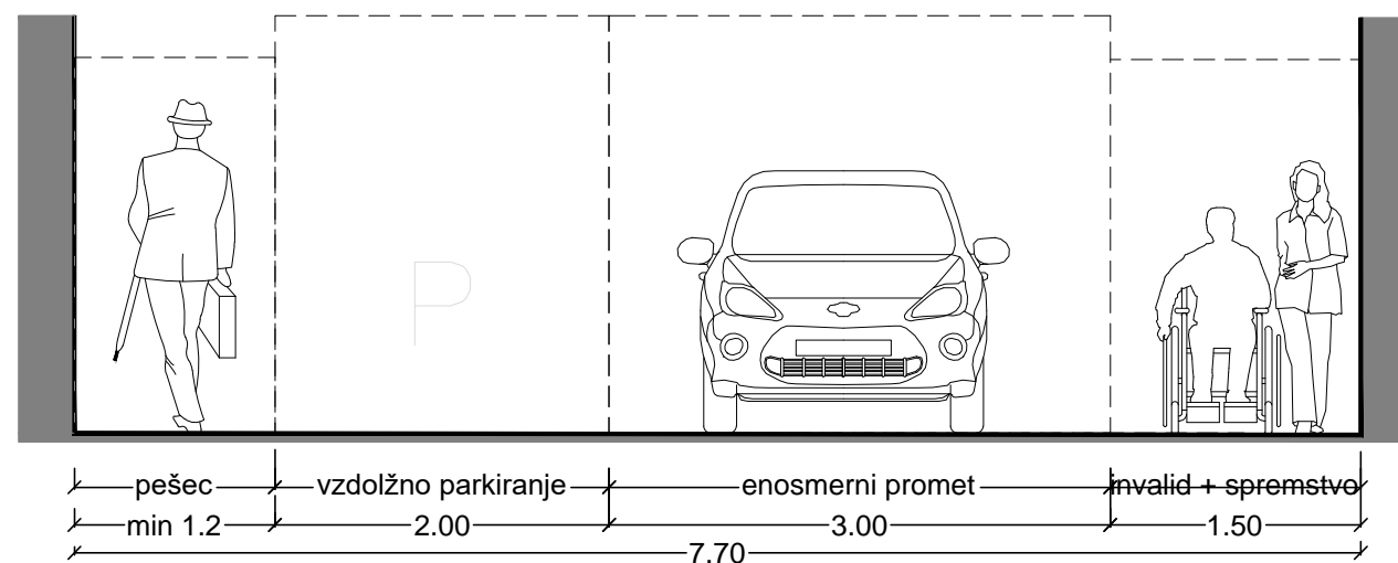
CESTNI PROFIL B-B STARA CESTA OD HIŠNE ŠT. 4 DO 28 IN OD 47 DO 52
